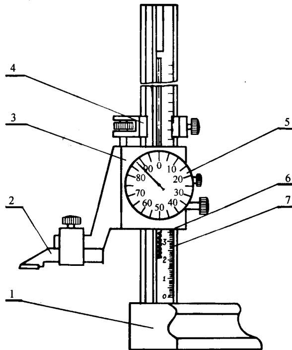
图3 圆标高度卡尺
