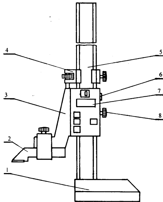
图2 电子数显高度卡尺
