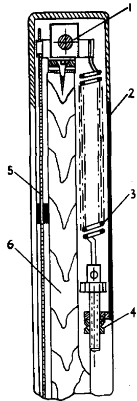
图 1 因瓦标尺结构示意图 1—等臂杠杆；2—盖板；3—弹簧； 4—张力调节螺母和固定螺母； 5—因瓦带；6—木质尺身
