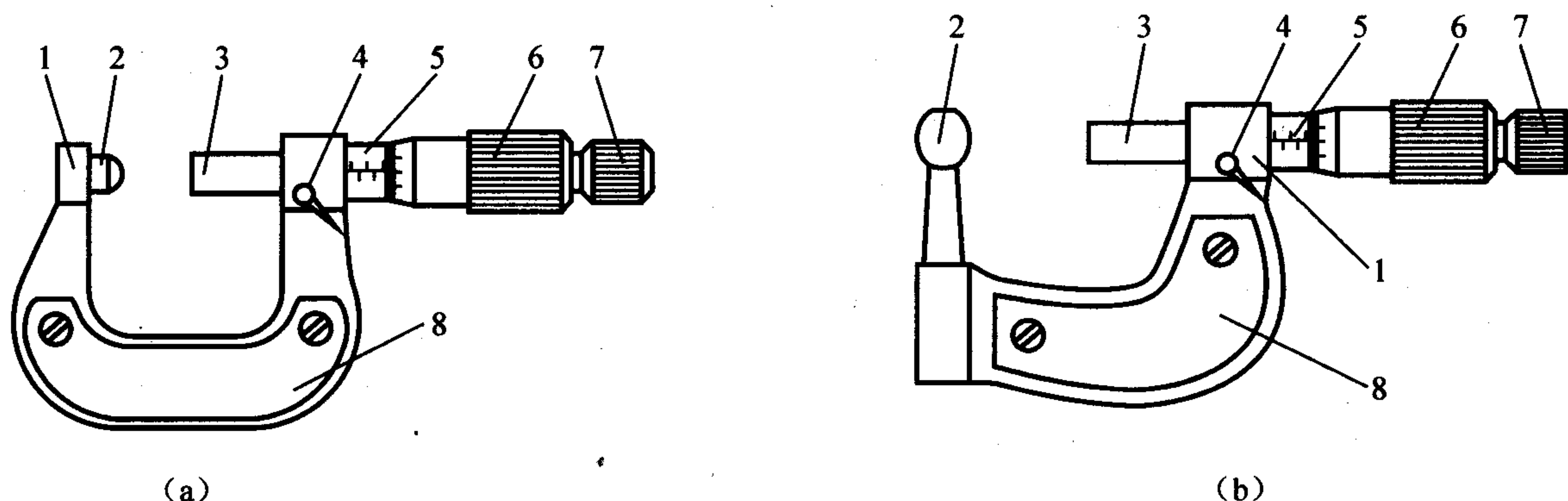
图4 壁厚千分尺
