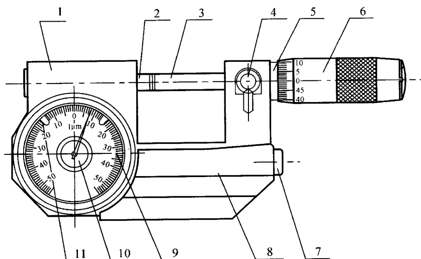
图1 杠杆千分尺
