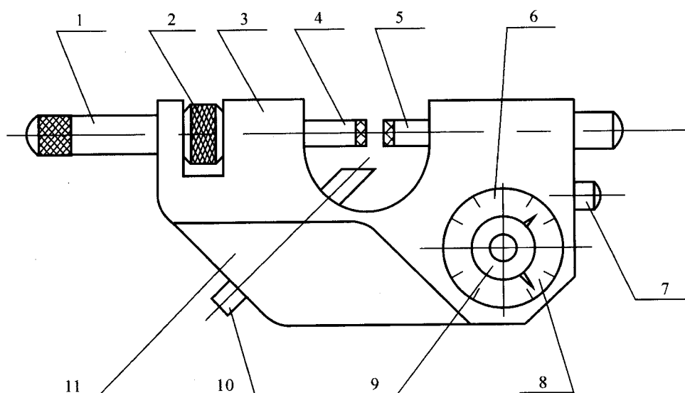
图2 杠杆卡规
