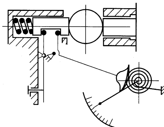
图3 杠杆传动机构
