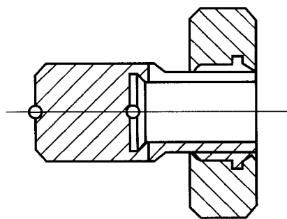
图 6 延长杆
