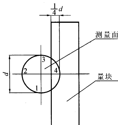
图 7 两测量面平行度检定的量块位置
