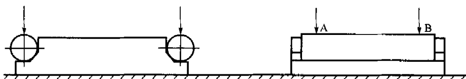
图6 两圆柱轴线的平行度测量位置示意图
