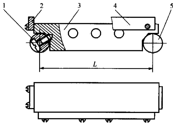
图 1 窄型正弦规
