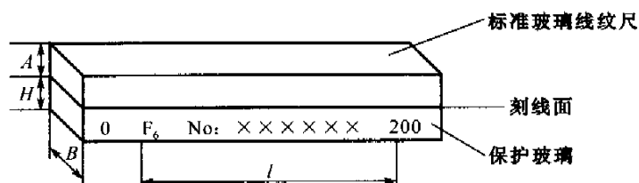
图 1 玻璃尺
