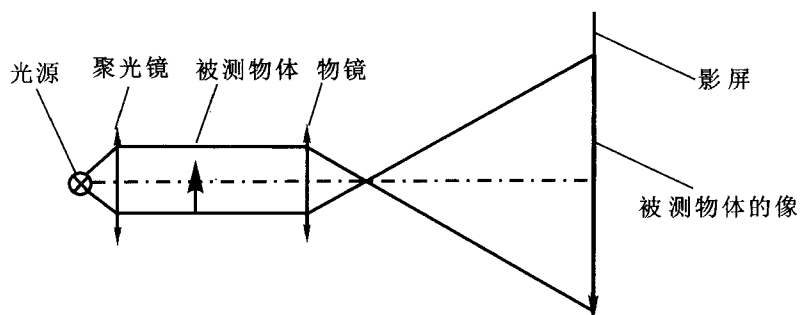
图3 工作原理图
